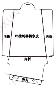
F6控制器挡水板-0523
