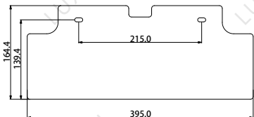
MHH控制器挡水皮 1210000003
