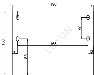
190-150挡水皮 -
