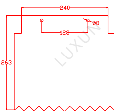
E8领跑版E-S电池盒挡水皮 1209000074
