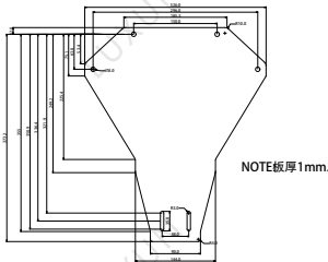
LX08-W挡水皮 1209000044
