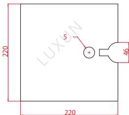
D9控制器挡水皮 1209000064
