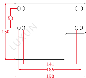
1号控制器挡水皮 1209000067
