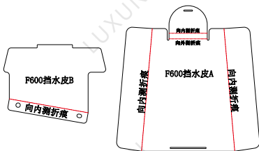
F600挡水板 1209000111
