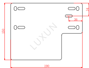
2号控制器挡水皮 1209000079
